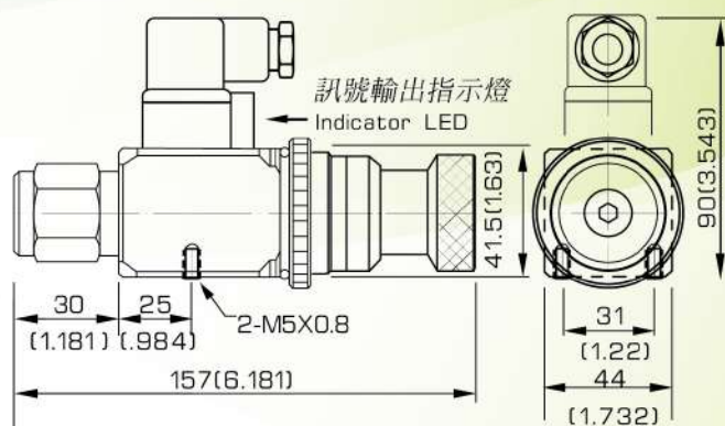
尺寸圖 / Dimension mm(inches)
