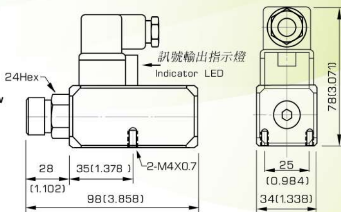
尺寸圖 / Dimension mm(inches)
