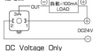
配電圖
