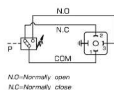
油電符號表 / Graphic Symbol
